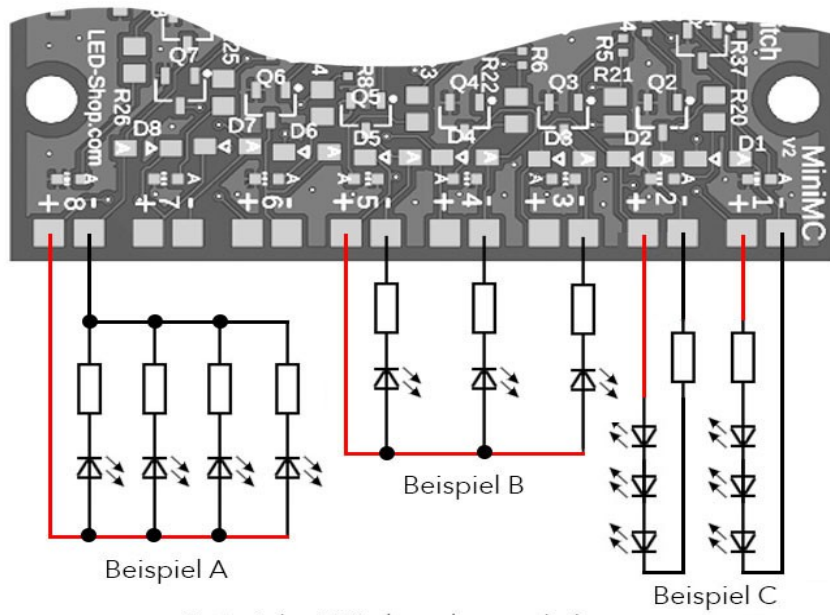
Beispiele: LEDs korrekt verschalten
